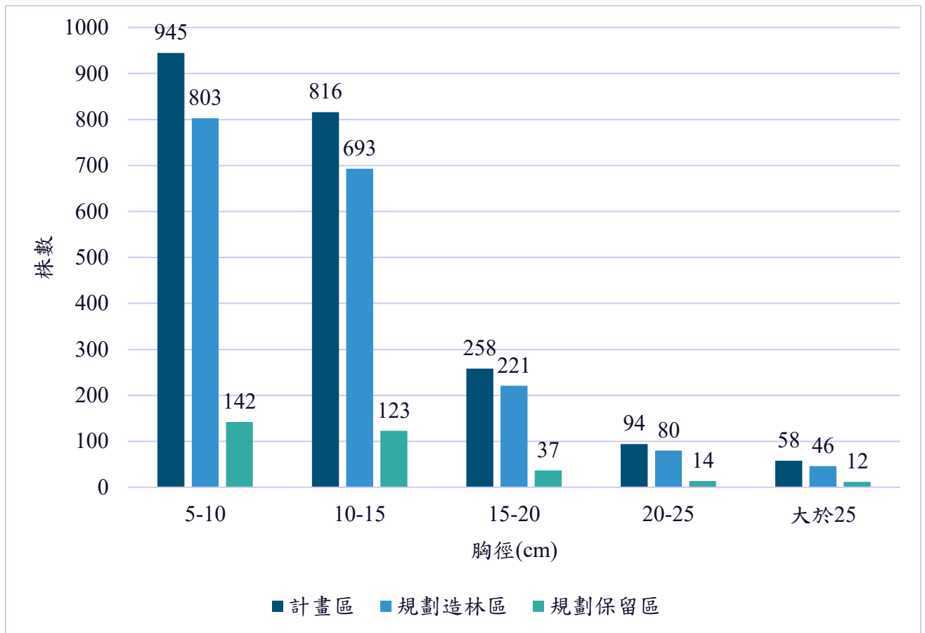
圖 11 計畫區、規劃造林區及規劃保留區之胸徑級分布情形
